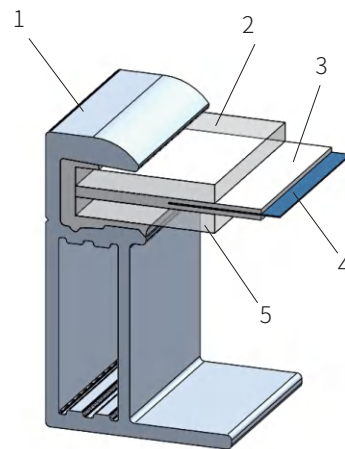
Tweezijdige modules (met frame)
